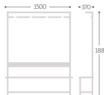
BFZP-1500 1.5MT
